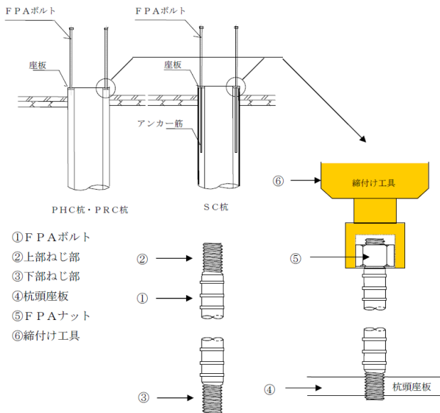
図1 FPA工法の構成
