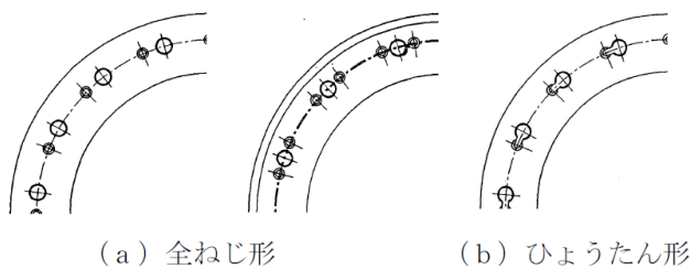
図2 ねじ穴形状タイプ
