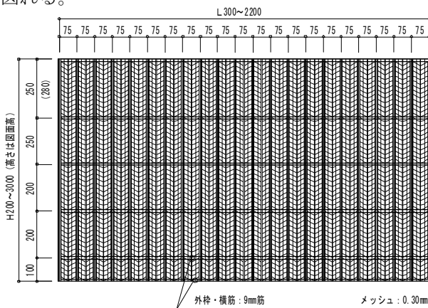
エコウェルメッシュ標準構造図
