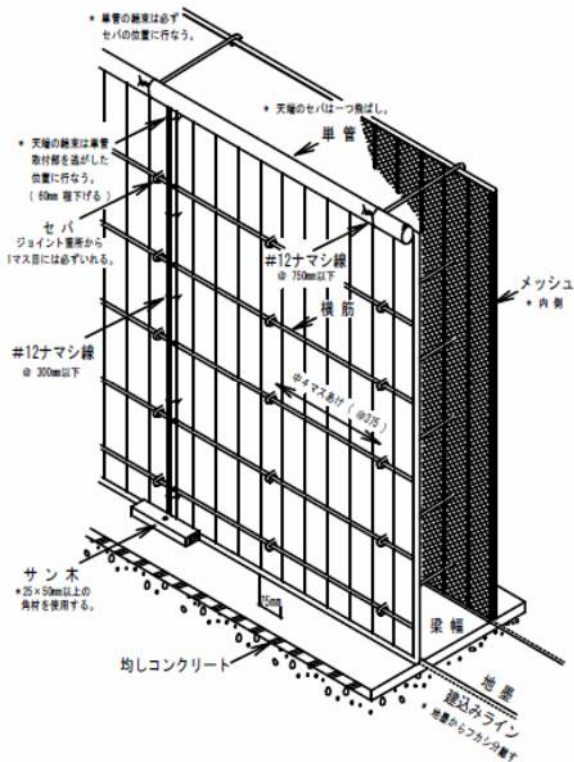
エコウェルメッシュ標準納まり図
