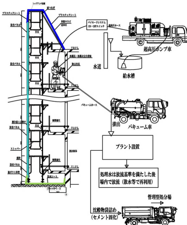
外壁部集じん装置付超高压水洗工法全体概略図
