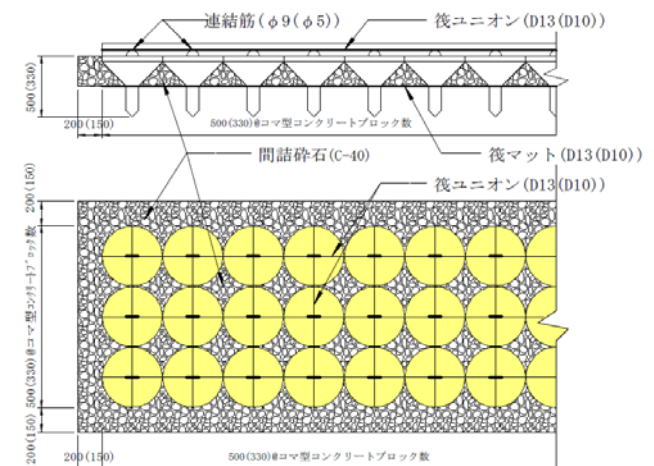
図1-1 トップベース工法構造断面及び平面
