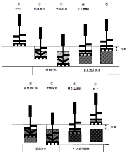
図1-5: 2サイクル施工手順略図
