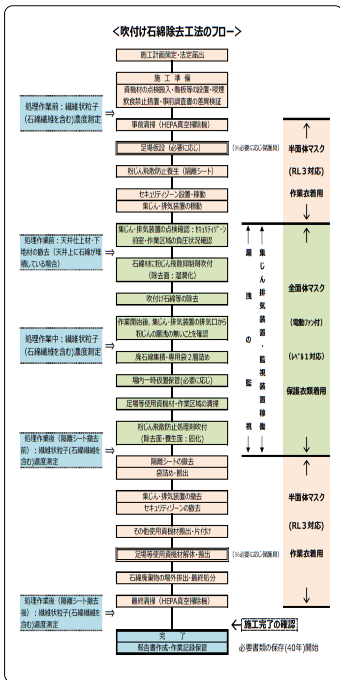
〔施工フロー図〕
