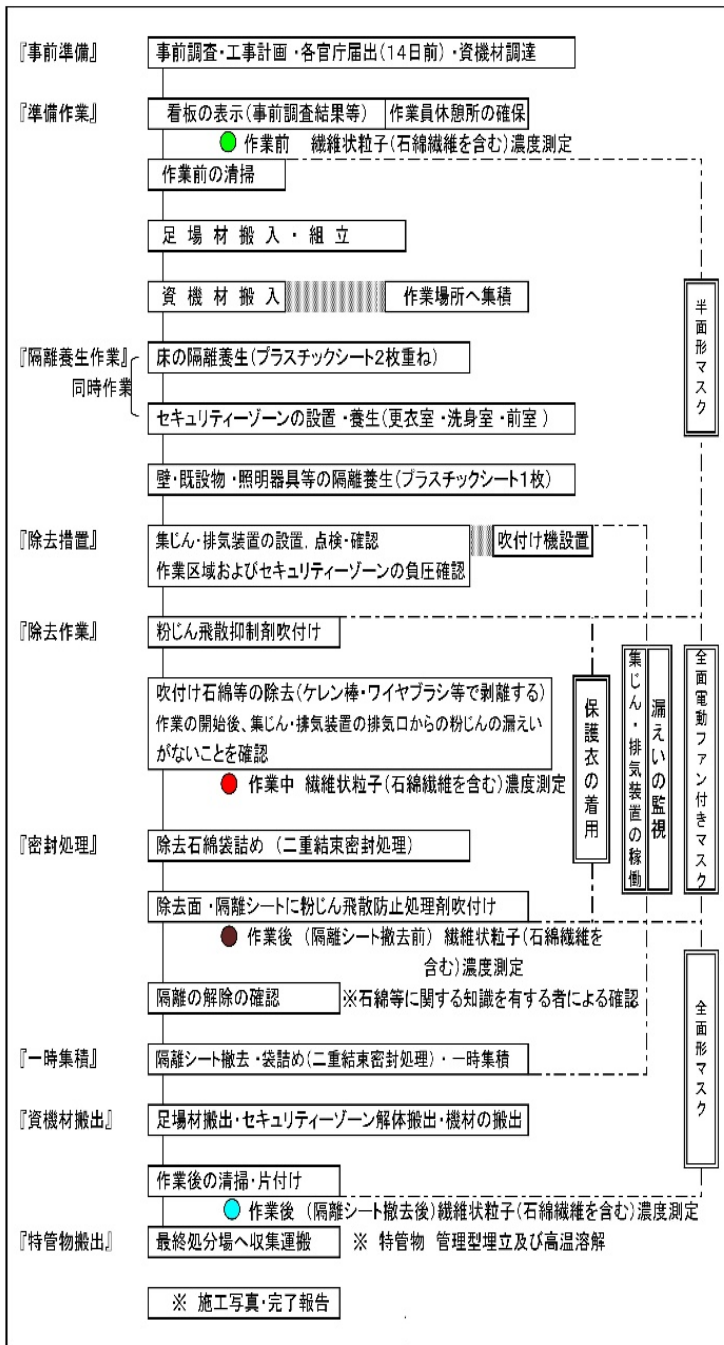
【施工フロー図】
