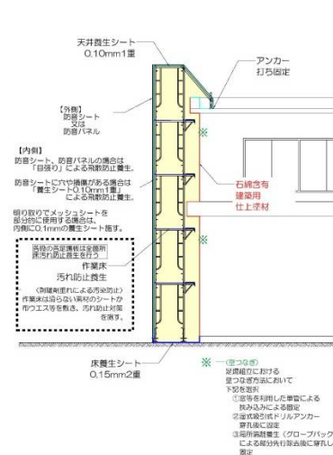
飛散防止養生計画【作業計画(案)】
